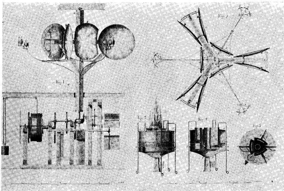
Fig. 33. Løwenørns spejlfyr set fra siden og fra oven. Nederst til højre olielamperne. Tavle i Løwenørns: Om Fyrers Indretning. Videnskabernes Selskabs Skrifter 1806.
