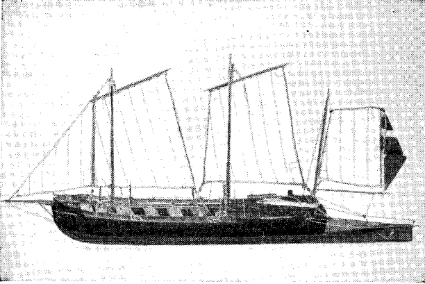
Fig. 41. Model af en kanonjolle fra 1809. Bemærk det lave agterskib. (Marinemuseet)
